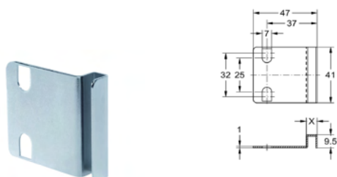
2549 Schließwinkel
