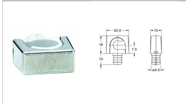
2442 Stangenführung
