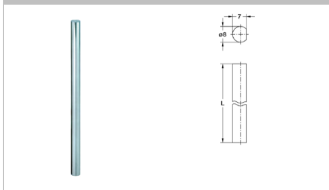
0087 Stange ø8
