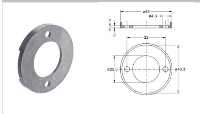
3006 Ausgleichsring
