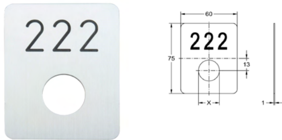
2116 Nummernschild
