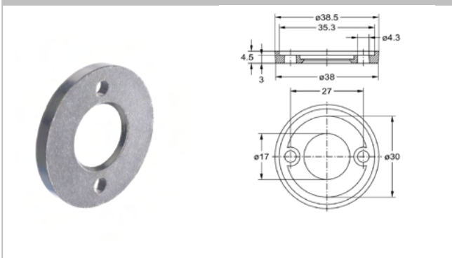
3005 Ausgleichsring
