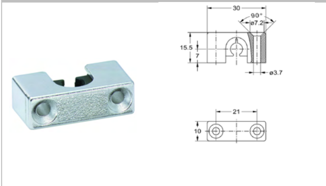
1311 Stangenführung
