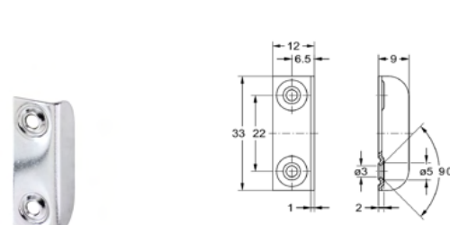
2572 Schließwinkel
