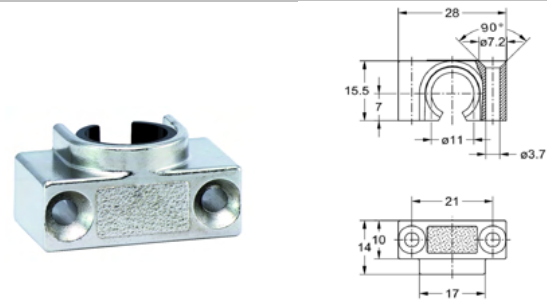
1310 Hakenlager
