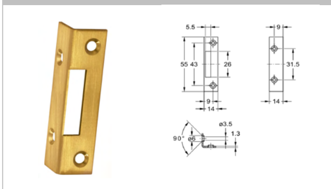
2591 Schließblech
