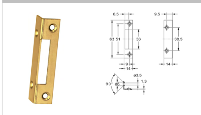
2596 Schließblech
