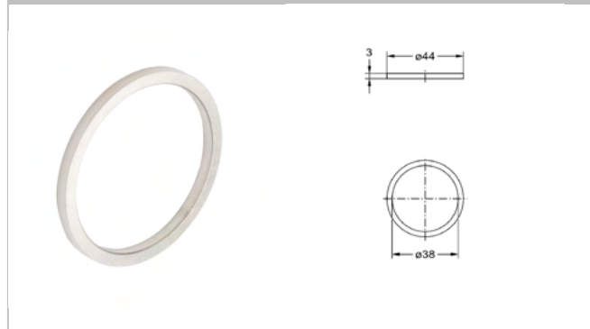
2618 Distanzscheibe
