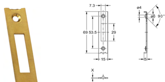
2585 Schließblech
