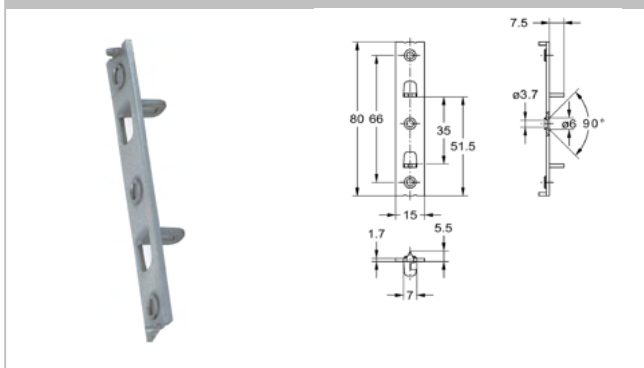
2524.25 Schließblech
