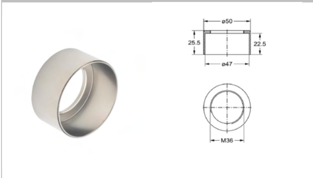
2617 Rohrmutter
