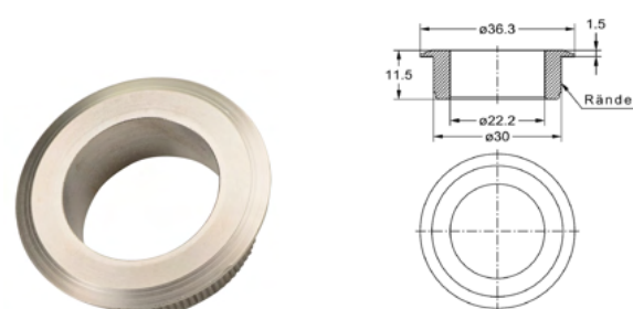
7430 Ausgleichsrosette
