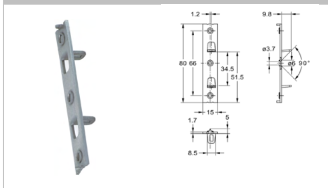
2524.30 Schließblech
