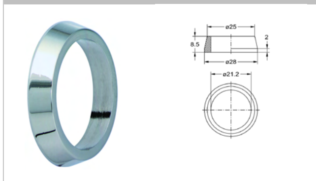
2920.08 Ausgleichsring
