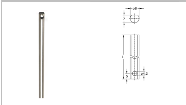
2363 Stangenführung
