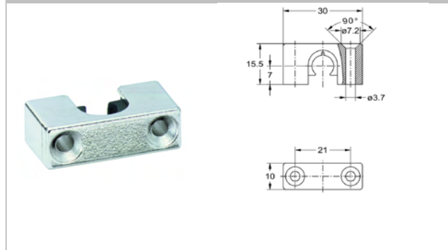
1312 Stangenführung
