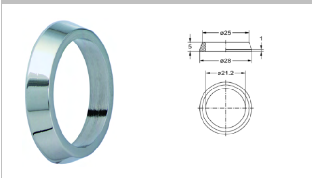
2920.05 Ausgleichsring
